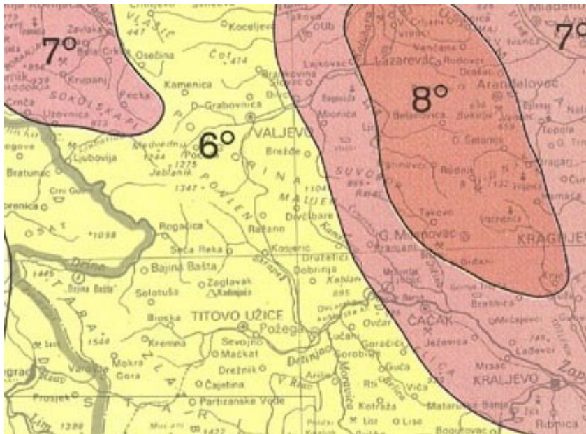
Сеизмолошка карта Србије
